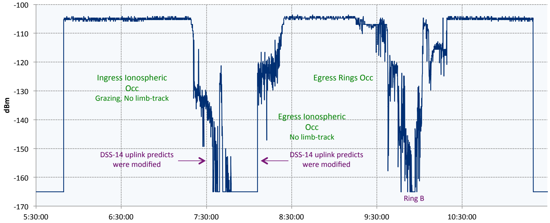
DSTRcvrAGCba (E-0216) vs SCET
