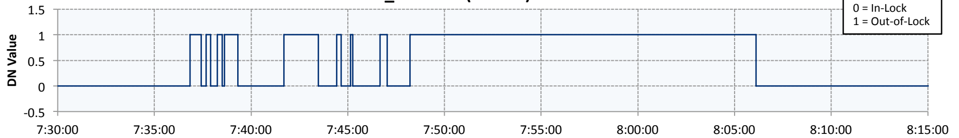
DST_UNLOCK (E-0418) vs SCET
