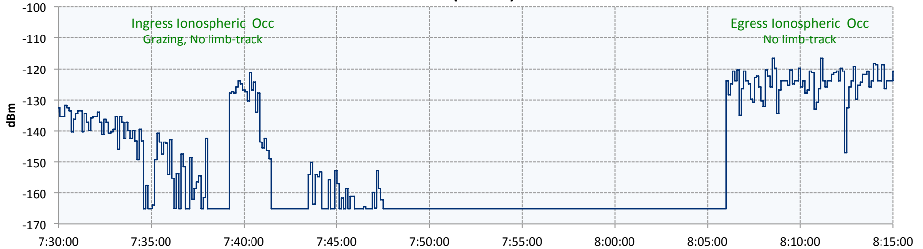
DSTRcvrAGCba (E-0216) vs SCET
